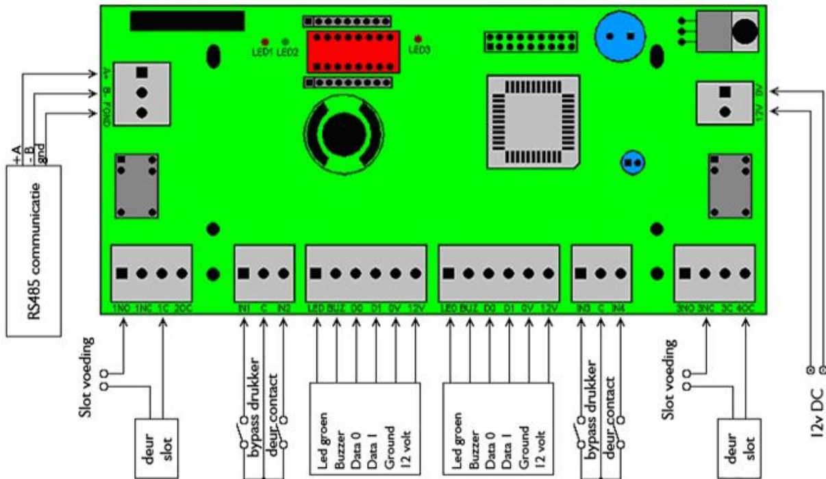
AXURC-PCB
