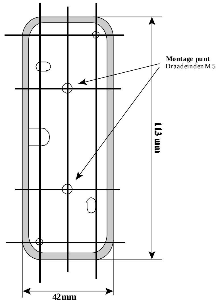
Grondplaat AXM-lezer
