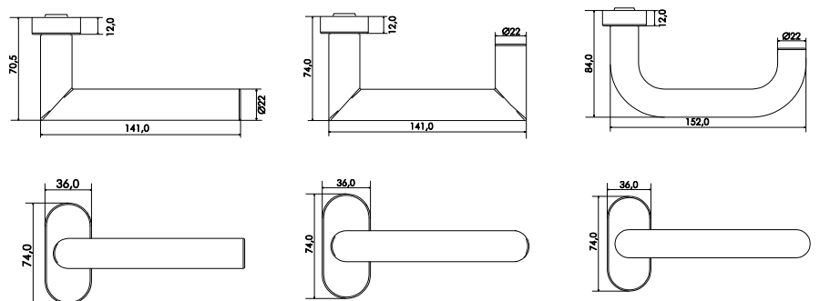
Ovalrosette Mechanikseite
