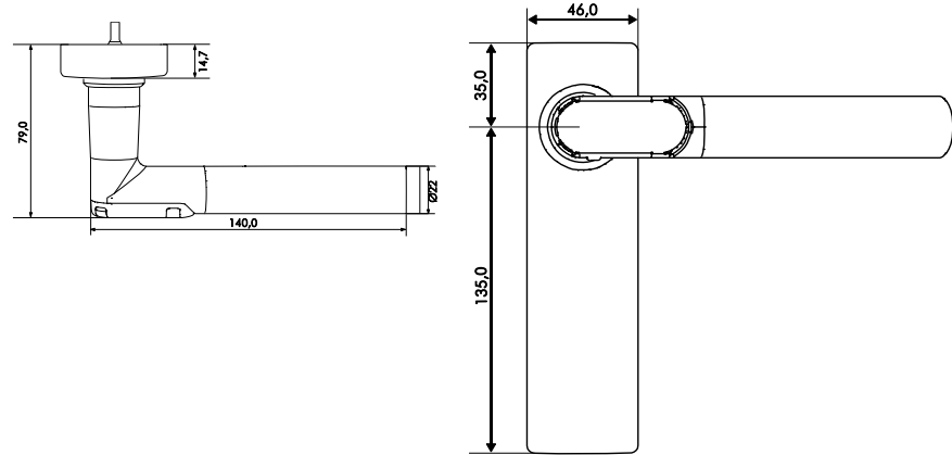
Kurzschild Elektronikseite
