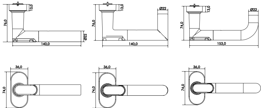
Ovalrosette Elektronikseite
