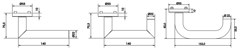
Rundrosette Mechanikseite und Drückervarianten
