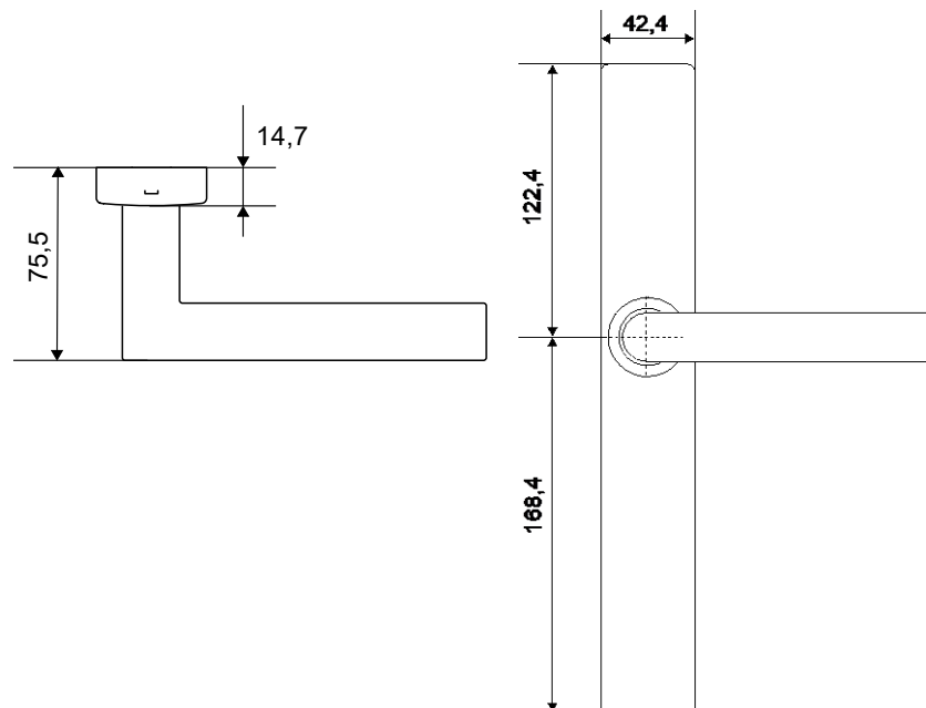
Langschild schmal Mechanikseite
