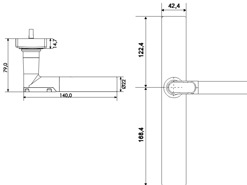
Langschild schmal Elektronikseite
