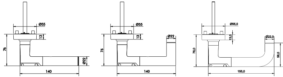
Rundrosette Elektronikseite und Drückervarianten
