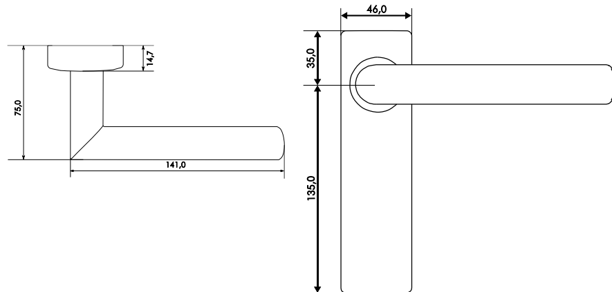
Kurzschild Mechanikseite
